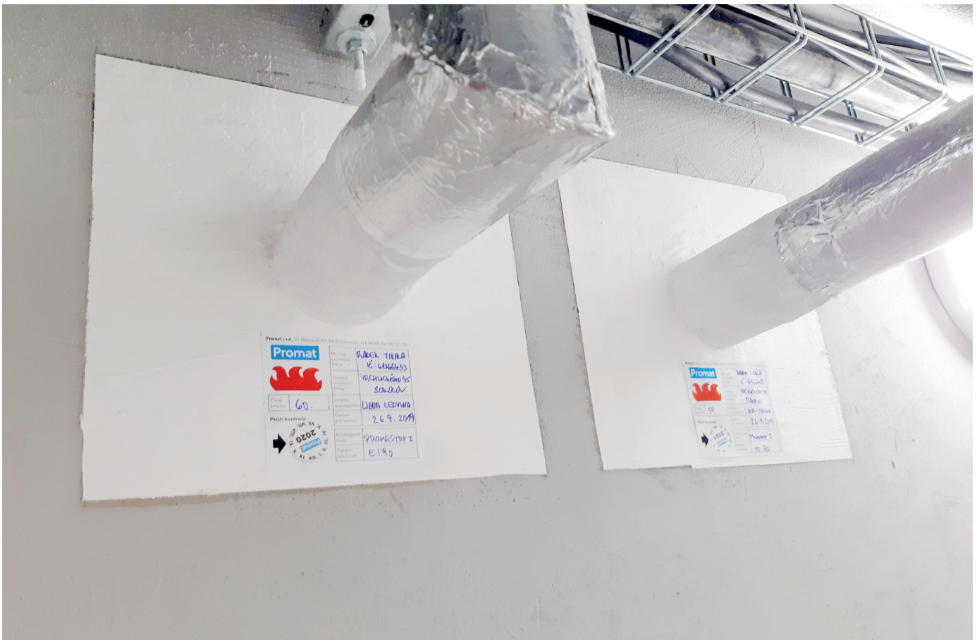
Prostup ocelového potrubí s nehořlavou izolací a stěrkou PROMASTOP®-I
