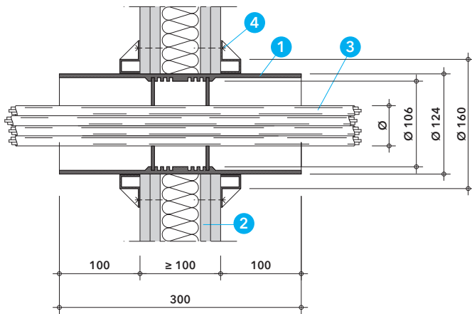
Detail A - prostop v lehké přičce
