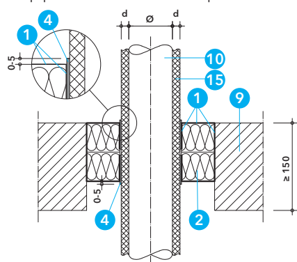
Detail W - prostup plastového izolovaného potrubí ve stropě 2)
