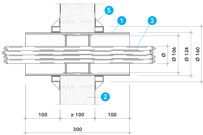
Detail B - prostop v masivní stěně
