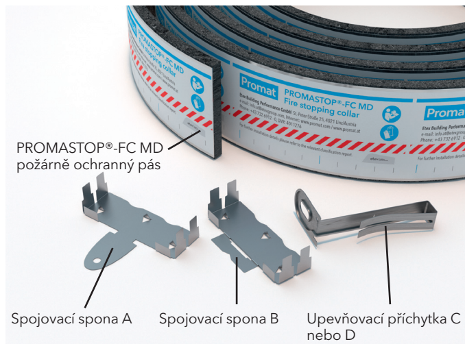
Detail J - spojovací spony a upevňovací příchytky
