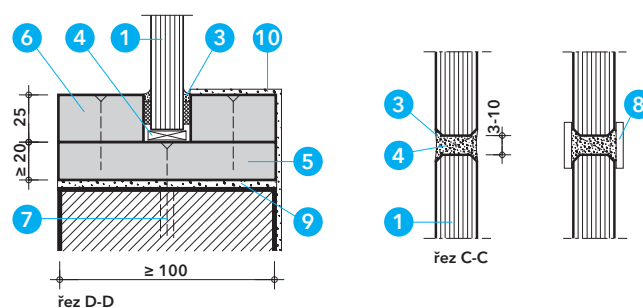
Detail C - připojení k podlaze
