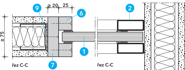
Detail E - připojení k lehkým příčkám
