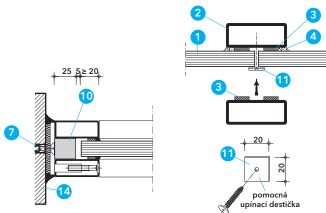
Detail B - vodorovný řez A-A
