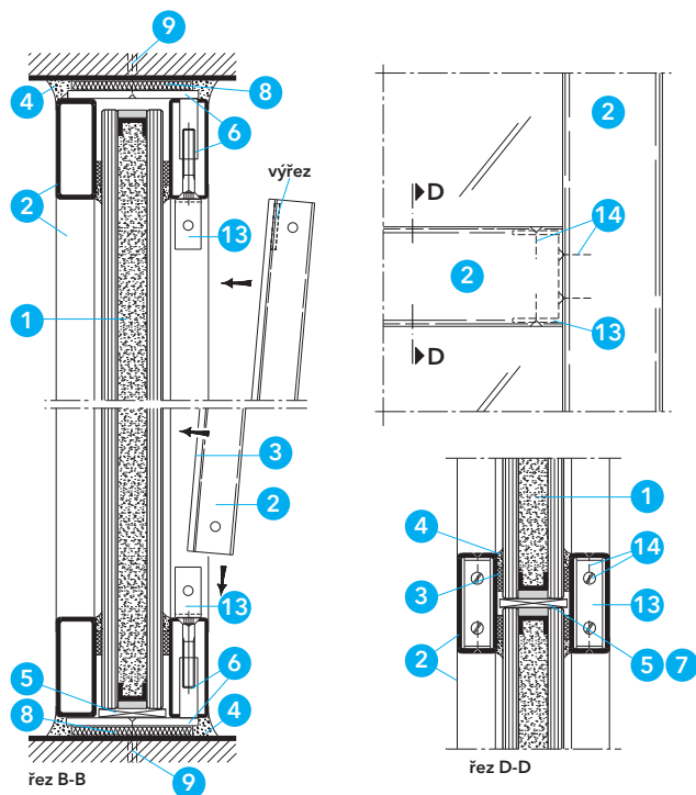
Detail F - svislý řez
