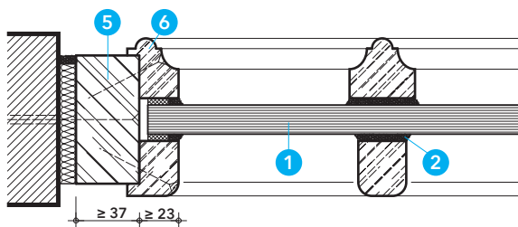
řez A-A
