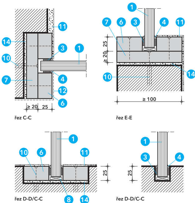
Detail D - připojení k masivní stěně
