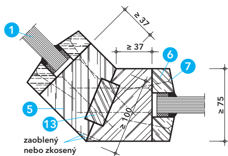
Detail E - rohové spojení > 90° až < 180° (≤ EI 45)
