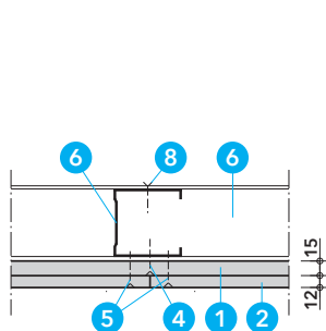
řez B-B
