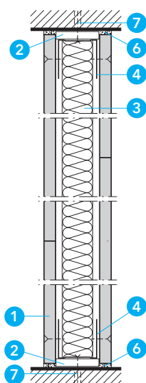
řez A-A
