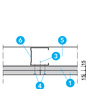
řez B-B
