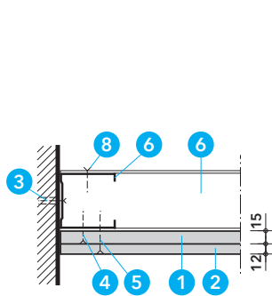
řez A-A
