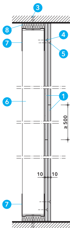
řez C-C
