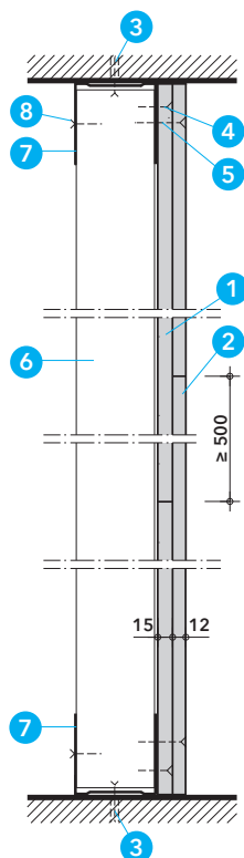
řez C-C
