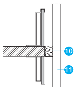
Detail D - požární utěsnění
