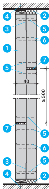
Detail B - připojení k podlaze a stropu
