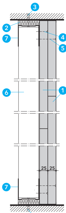
řez C-C
