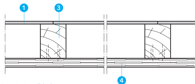
Dřevěný podhled
