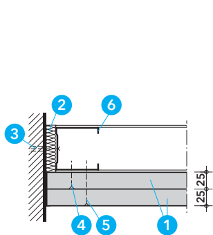
Detail A - pohled
