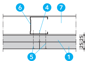
řez B-B
