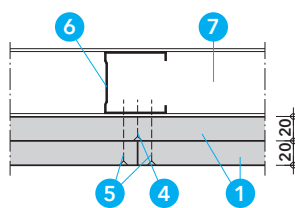
řez B-B
