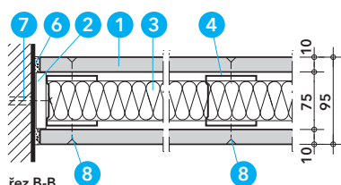
Detail C - vodorovný řez
