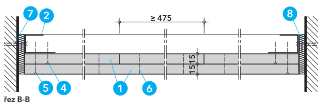
Detail C - vodorovný řez
