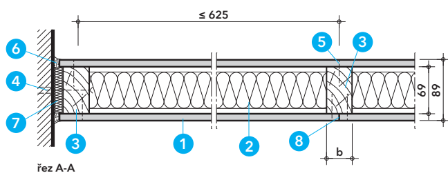
Detail B - vodorovný řez
