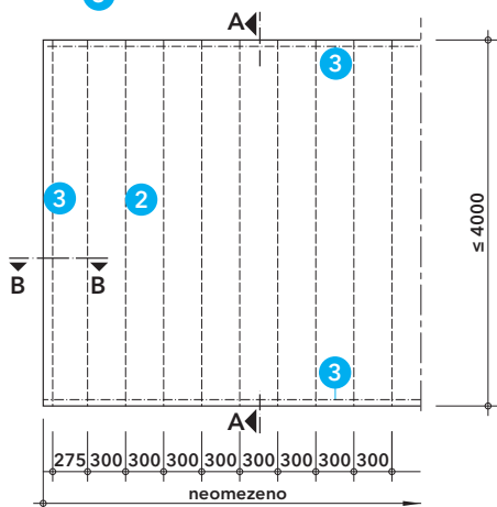
Detail A - schéma
