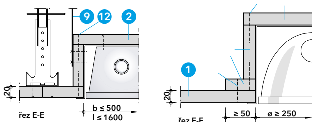
Detail F - vestavěné světlo
