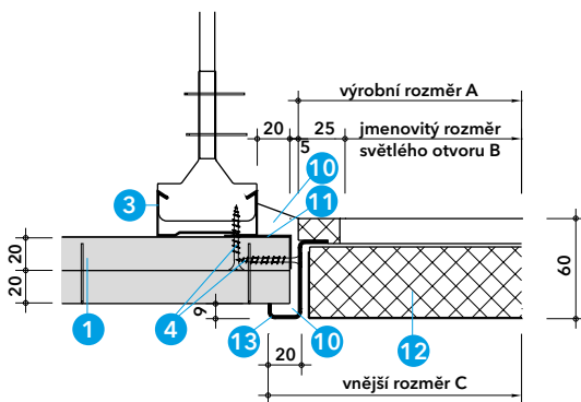
Detail C - revizní dvířka Promat®, typ SP
